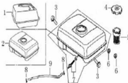
TANQUE DE COMBUSTIBLE
