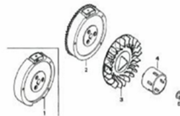
VOLANTE
