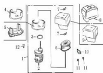
FILTRO DE AIRE
