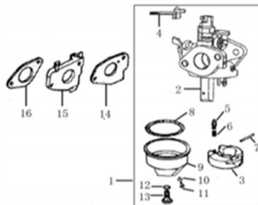
CARBURADOR
